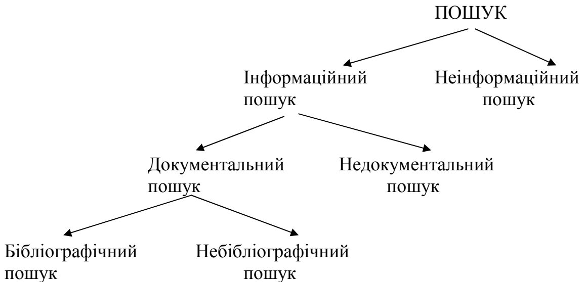
Рис.3.3. Дихотомічна класифікація пошуку
