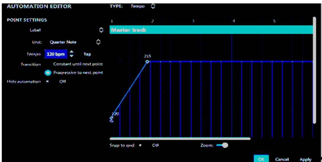
Рис.5. Вікно редагування
