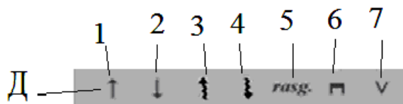
Рис. 38. Лінійка Д
