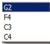
Рис. 21. Список ключів
